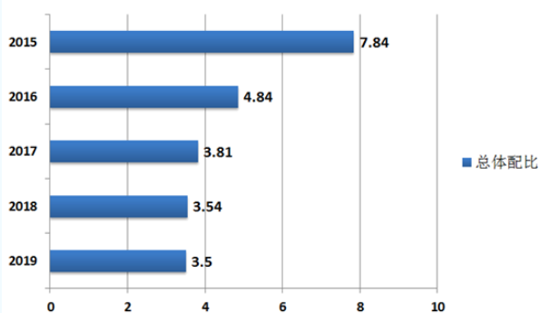
图1：2015-2019年新能源汽车充电桩配比情况
